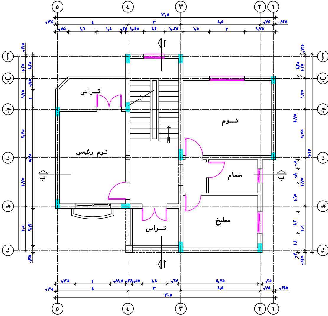
مسقط أفقى للدور الأول
