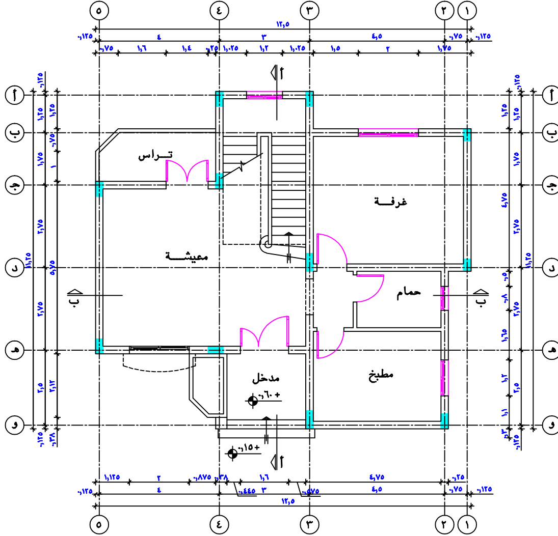
مسقط أفقى للدور الأرضى
